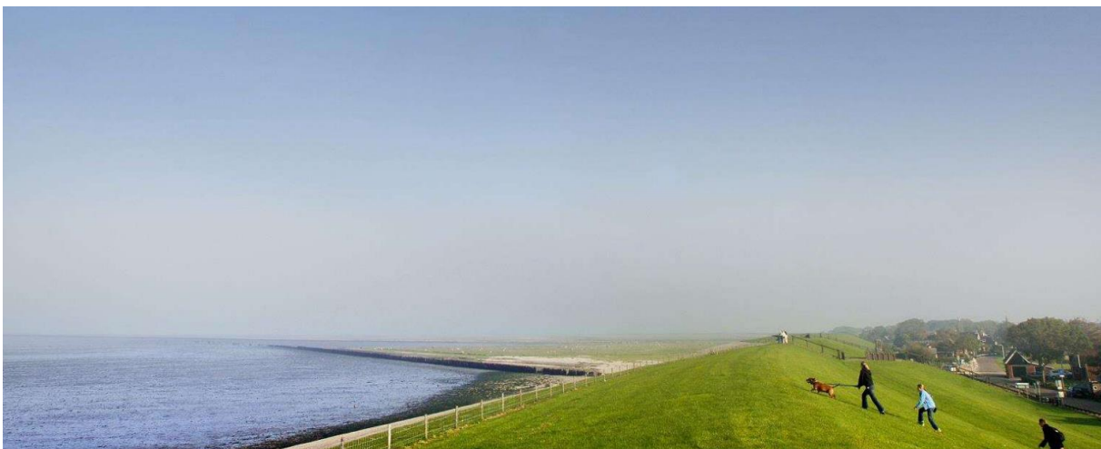
Bron: 1DYK
